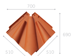
Meia Telha
